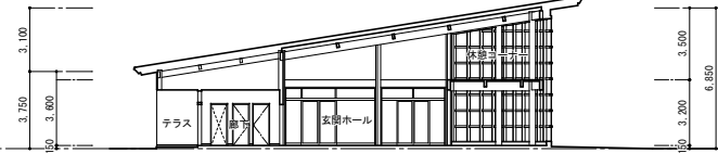
B～B断面図
