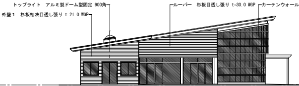
南立面図
