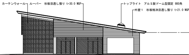
北面図
