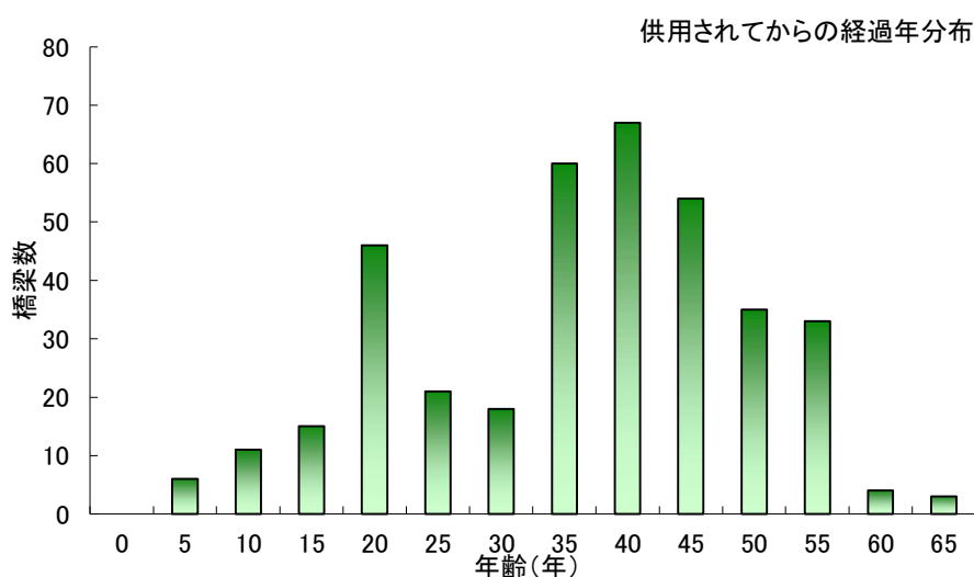
図 6 経過年の分布
