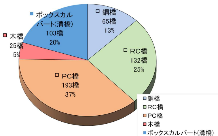
図 3 橋種別の橋梁数（径間数）
