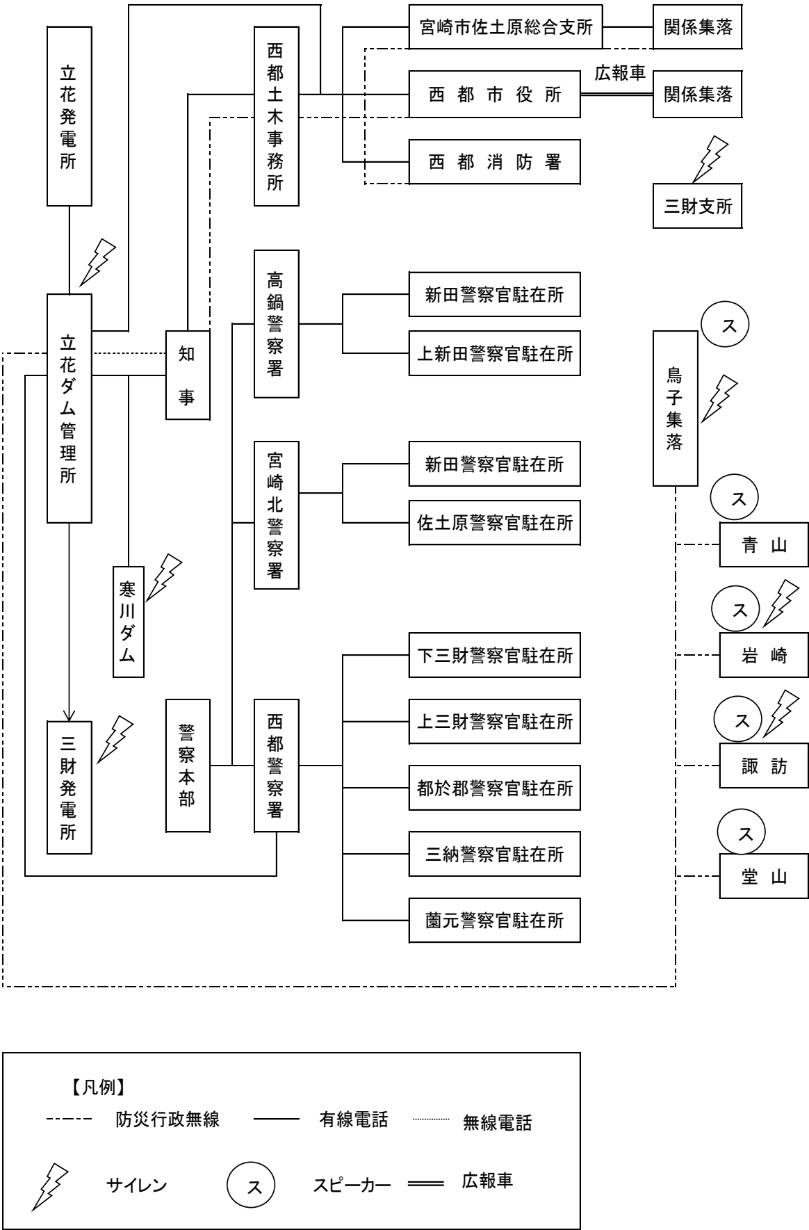
資料－４４ 三財川立花ダム放流開始時の通報系統図
